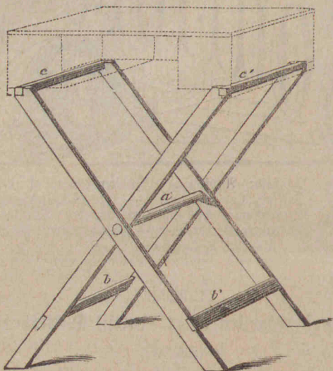
Træbuk, til Opstilling af Dukketheatret.
