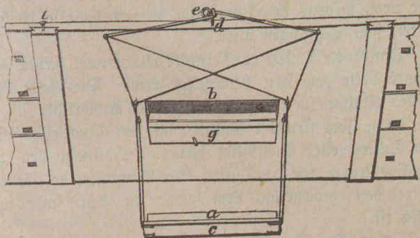
Den bevægelige Lem, set fra nedden. (g, den faste Lem, aabnet.)
