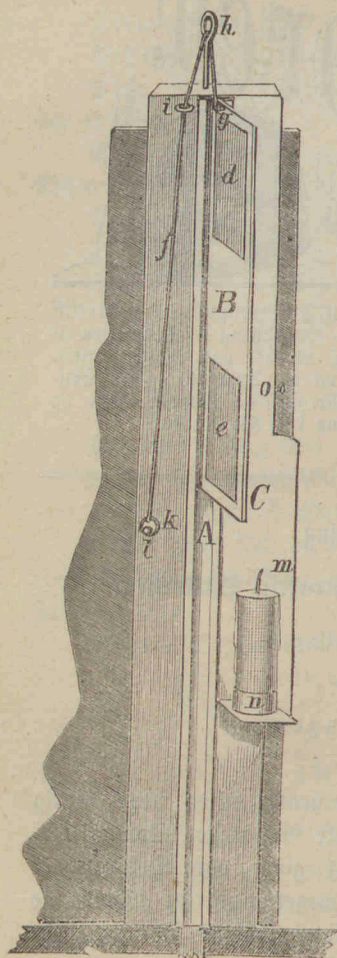
Et Belysningsapparat anbragt paa en af de faste Coulisjer tilhøjre.
