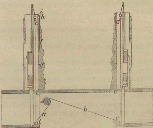
Snoreindretning til Ophængement af Vælsningen, vist paa to Coulisjer, (set bagfra).
