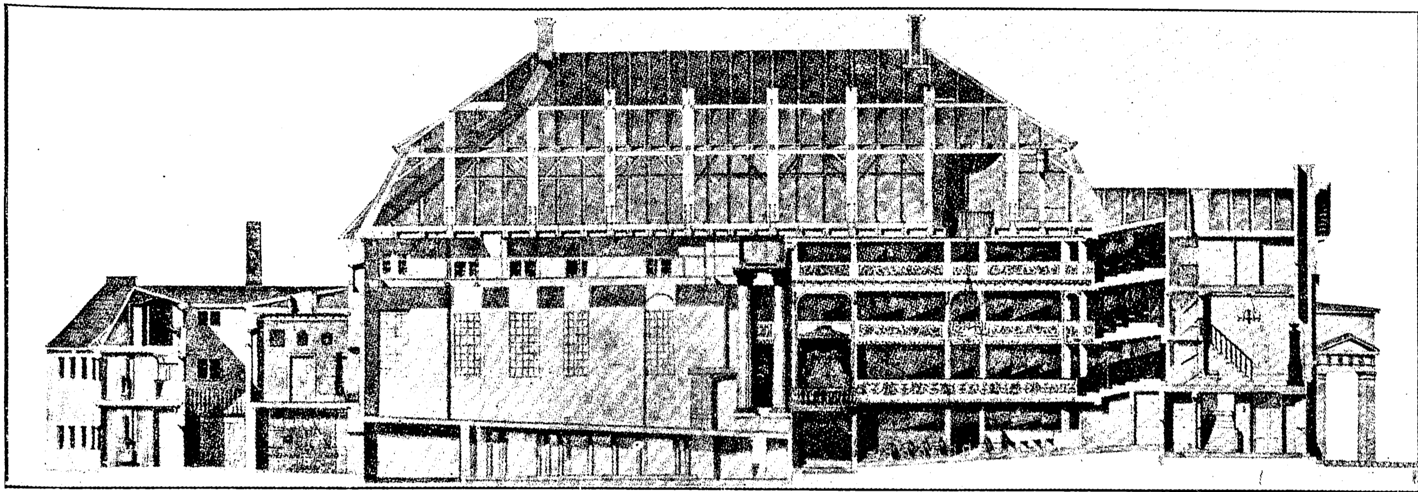
Længdesnit af Theaterbygningen 1792, efter Harsdorffs Tegning.
