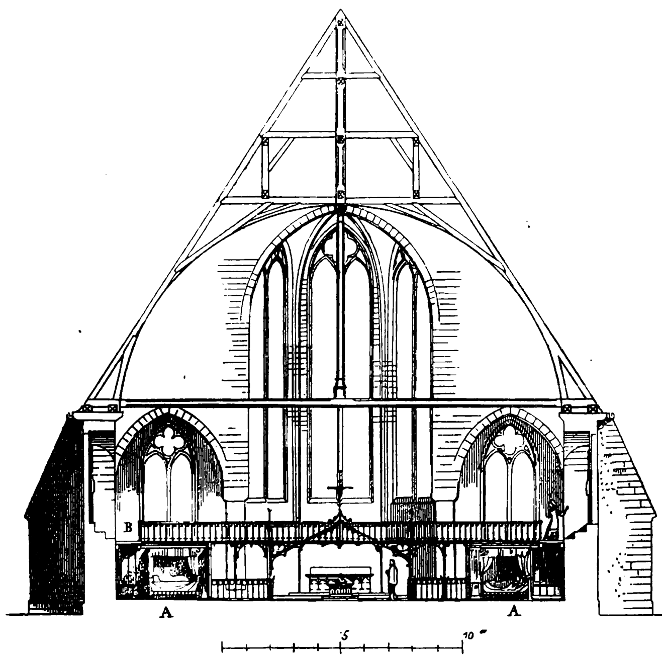
Fig. 7. Hospitalet i Tonnerre. Tværsnit af Salen. A. Alkove. B. Galleri. Efter Viollet le Duc VI, 111.
