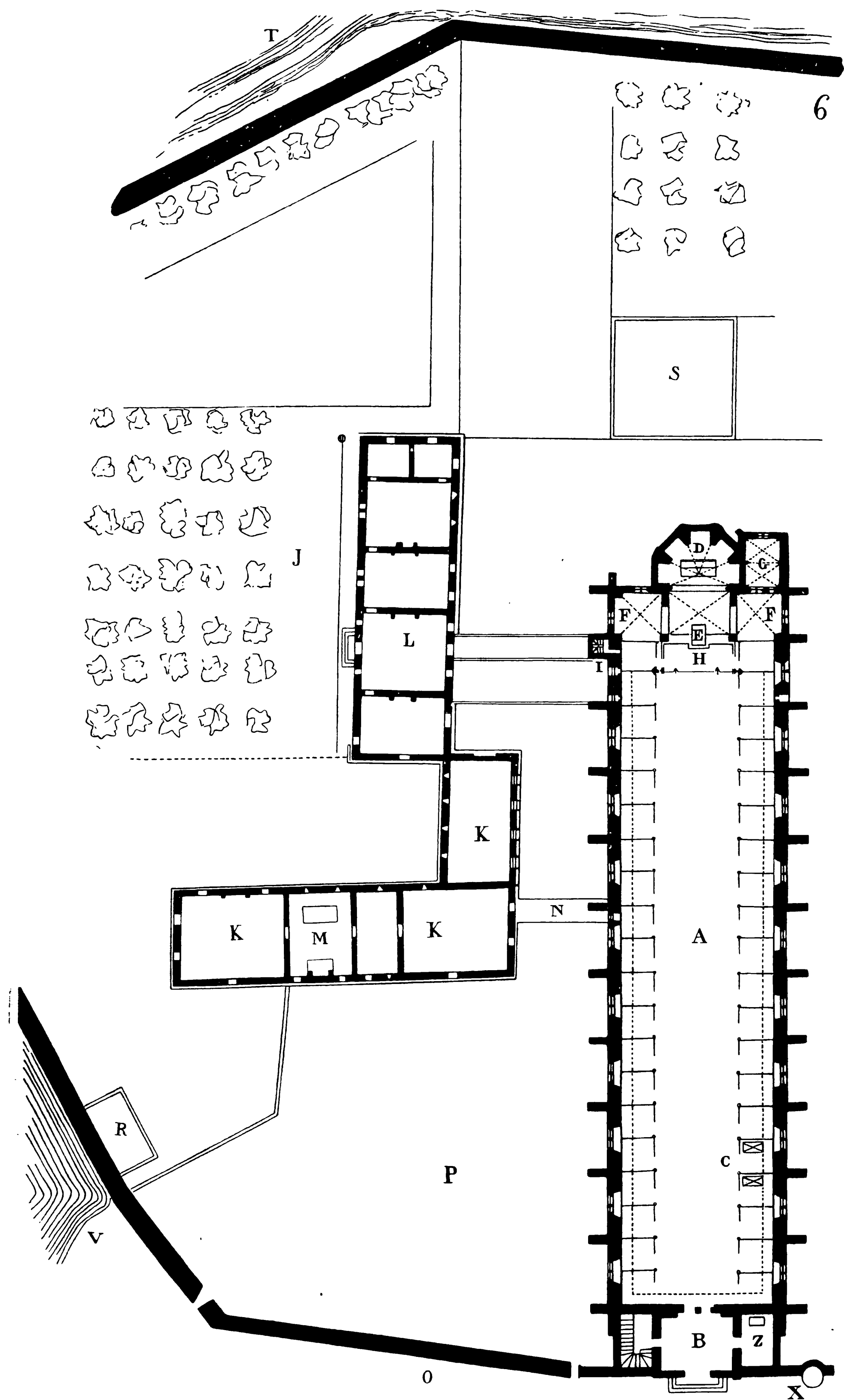
Fig. 8. Helligaandshospitalet i Tonnerre. Grundplan. Efter Viollet le Duc VI, 110.
